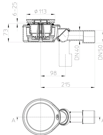
Schnitt A-A
